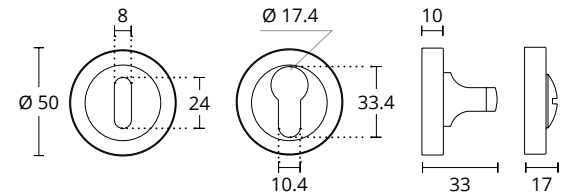
AF ΡΟΖΕΤΑ ΜΠΑΝΙΟΥ TURN & RELEASE ESCUTHEON
