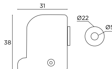
ΔΙΑΣΤΑΣΕΙΣ/DIMENSIONS
